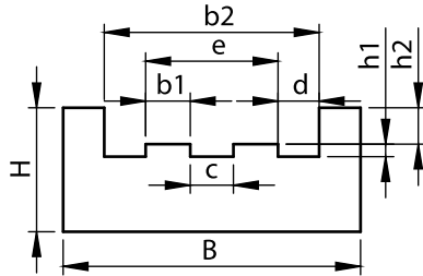
TK2 MODELİ ZİNCİR KIZAĞI
