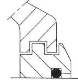
TS-U Keçe, TS5xxU
