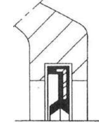
U-LOK Keçe, U5xx
