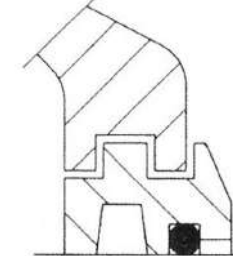
TS-UF Keçe, TS5xxUF
