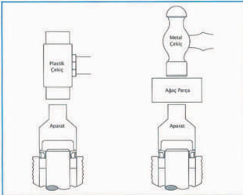
Şekil 16: Montaj Örneği
