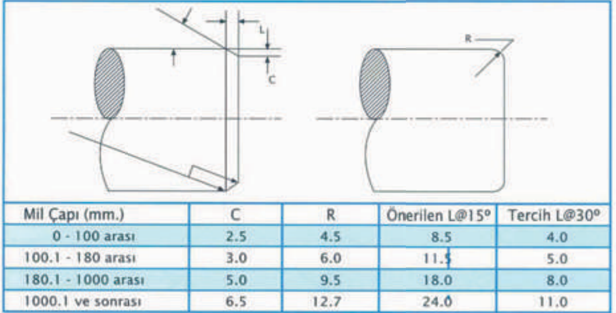
Şekil 5: Mil Dizaynı
