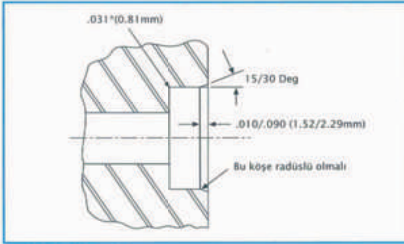
Şekil 4: Yuva Dizaynı
