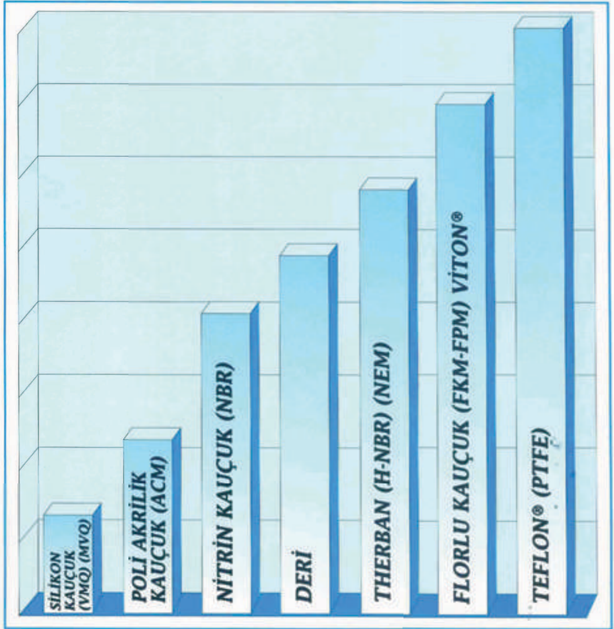
Şekil 2: Yağ Keçesi dudak malzemelerinin aşınma dayanıklılık mukayesesi
