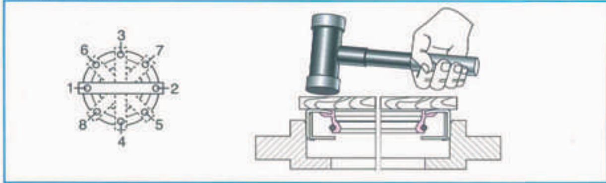
Şekil 11: Montaj Örneği
