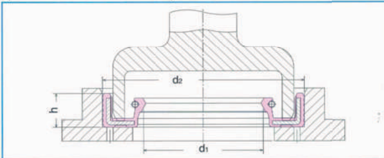
Şekil 6: Montaj Örneği
