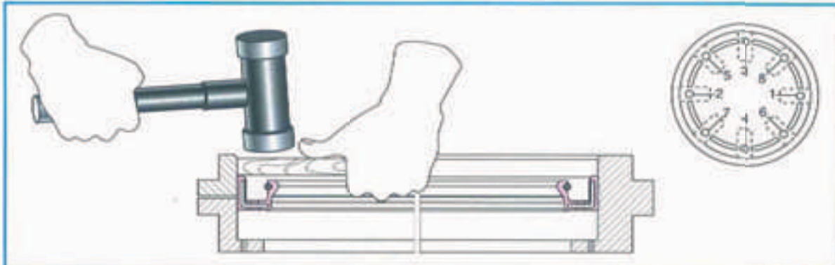
Şekil 12: Montaj Örneği
