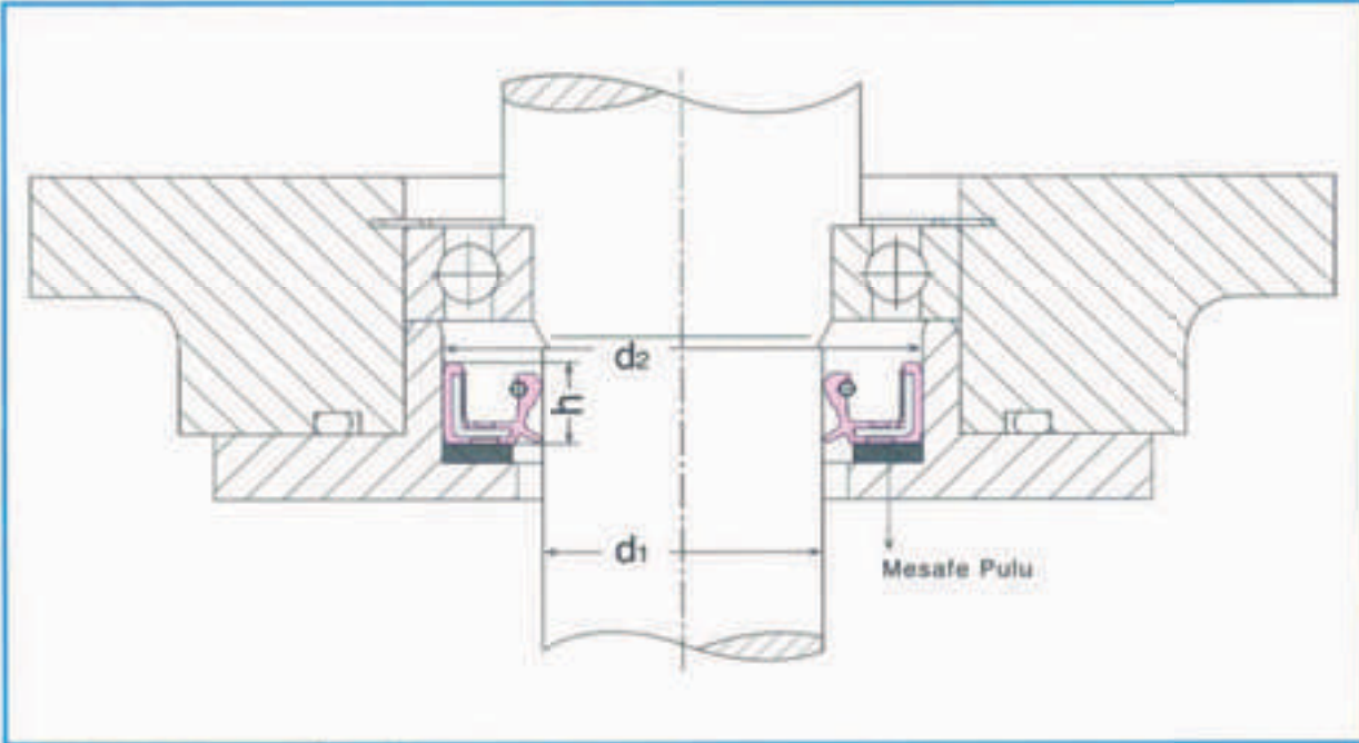
Şekil 15: Montaj Örneği
