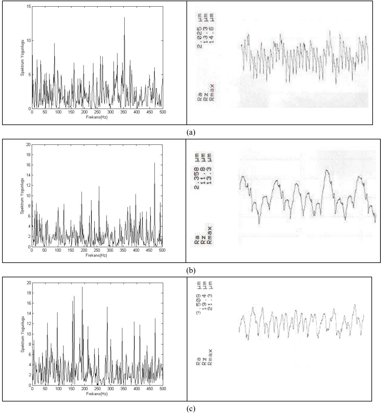
Şekil 2. Yaklaşma açısı ve talaş açısı değişimlerin pürüzlülüğe etkileri
