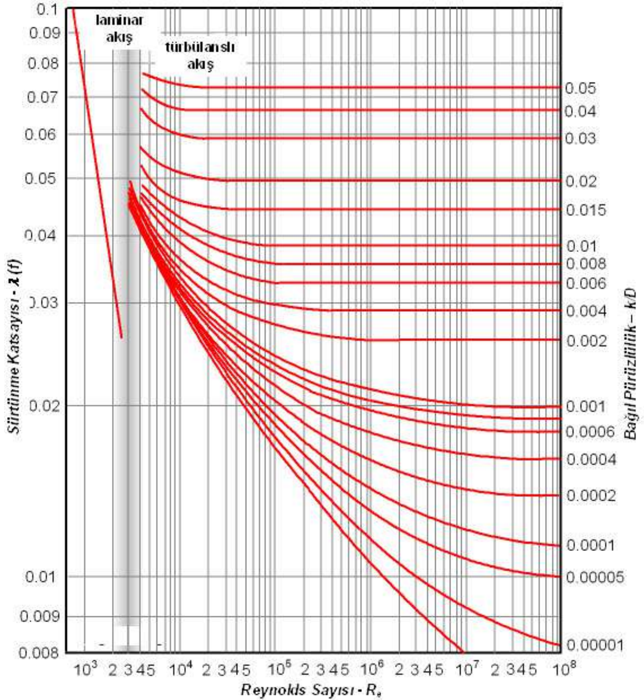
Şekil 1.2 Moody Diyagramı
