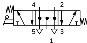
5/3 kol kumandalı yay merkezlemeli, H merkezli
