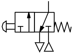
3/2 buton kumandalı, yay geri dönüşlü NK
