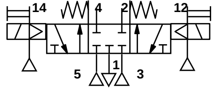
5/3 çift solenoid kumandalı (manuel kontrollü) Yay merkezlemeli kapalı orta konumlu
