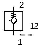
İkazlı çek valf
