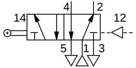
5/2 makaralı, hava uyarımlı Sınır anahtarı 1-2 ye açık
