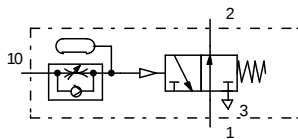
Pnömatik zamanlayıcı NA
