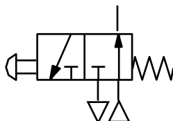
3/2 buton kumandalı, yay geri dönüşlü NA
