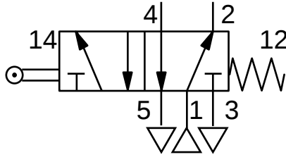
5/2 makaralı Sınır anahtarı 1-2 ye açık
