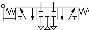
5/3 kol kumandalı yay merkezlemeli, merkezi kapalı
