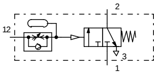
Pnömatik zamanlayıcı NK
