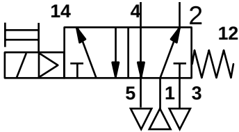
5/2 tek pilot solenoid kumandalı (manuel kontrollü) yay geri dönüşlü 1-2 ye açık
