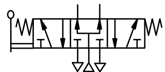
5/3 kol kumandalı yay merkezlemeli 1- 2ve 4'e açık
