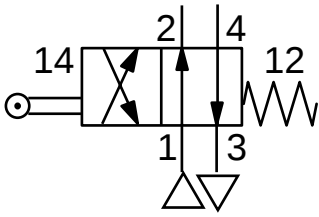
4/2 makaralı Sınır anahtarı 1-2 ye açık
