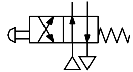
4/2 buton kumandalı, yay geri dönüşlü 1 4 e açık
