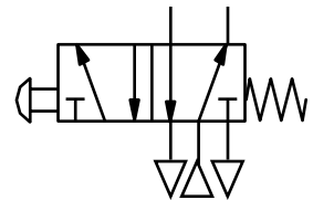
5/2 buton kumandalı, yay geri dönüşlü 1 2 ye açık
