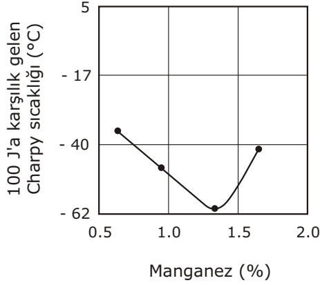
Şekil-7 Düşük Alaşımlı Çeliklerde Kaynak Metalinin Manganez İçeriği İle Çentik Darbe Tokluğu Arasındaki İlişki
