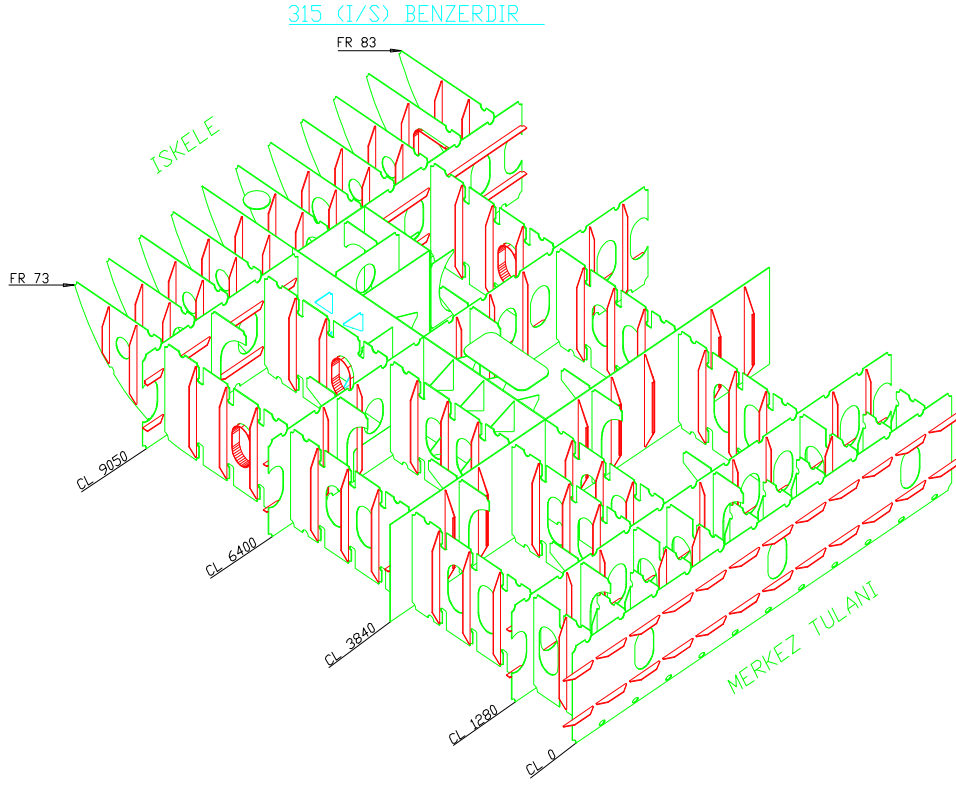
Şekil 1.2: Double bottom bloğu izometrik montaj resmi
