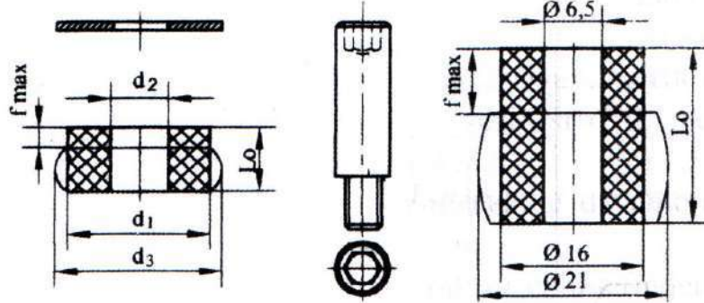
Şekil 2.8: Kauçuk yaylar
