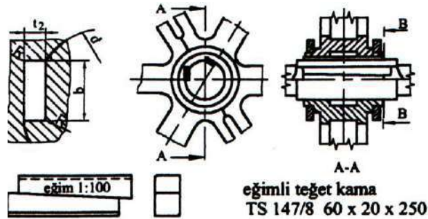
Şekil 1.8: Eğimli teğet kama ve uygulama örneği
