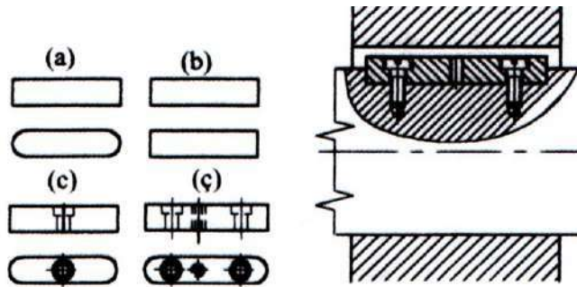
Şekil 1.11: Eğimsiz (Paralel yüzeyli) ince kamalar
