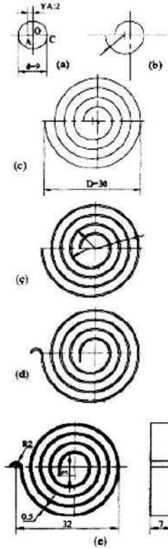
Şekil 2.18: Spiral yay çizimi
