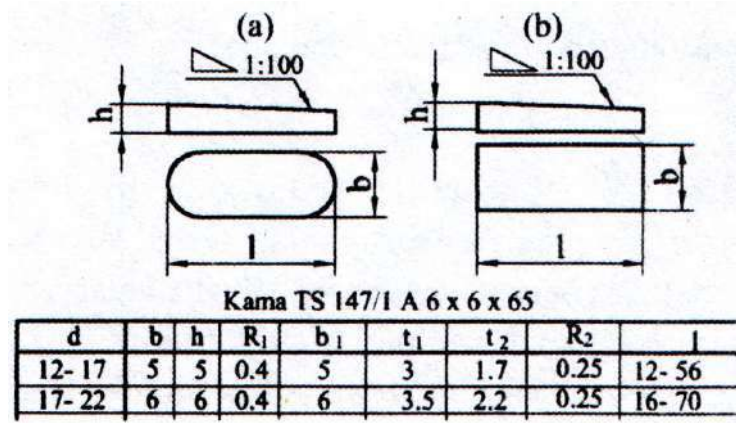
Şekil 1.15: Eğimli kama standart çizelgesinin incelenmesi
