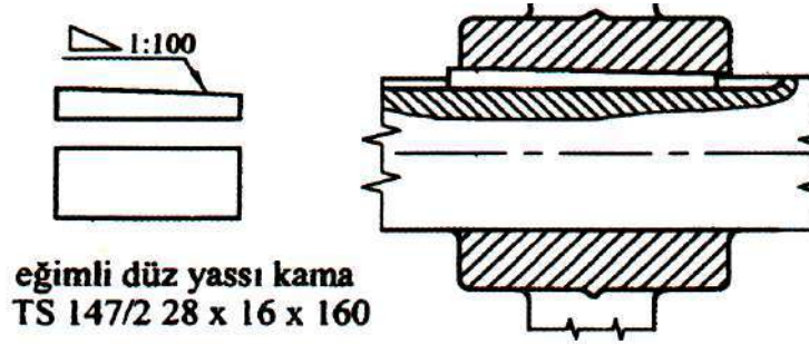
Şekil 1.3: Eğimli düz yassı kama ve uygulama örneği
