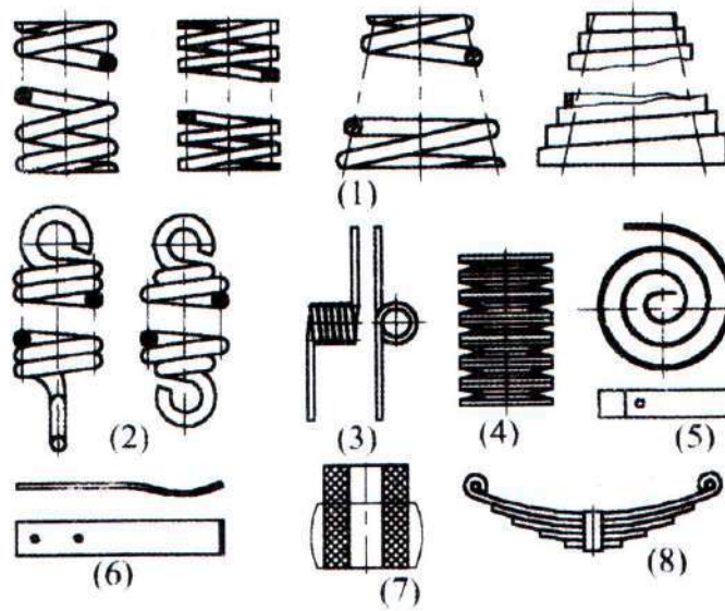
Şekil 2.1: Yay çeşitleri
