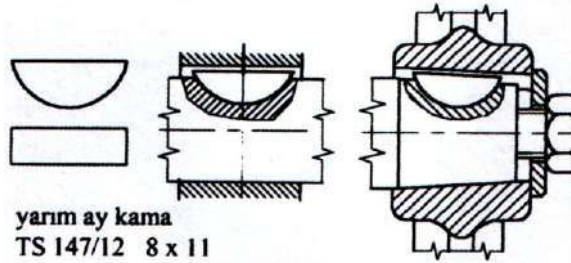
Şekil 1.13: Yarım ay kama ve uygulama örneği
