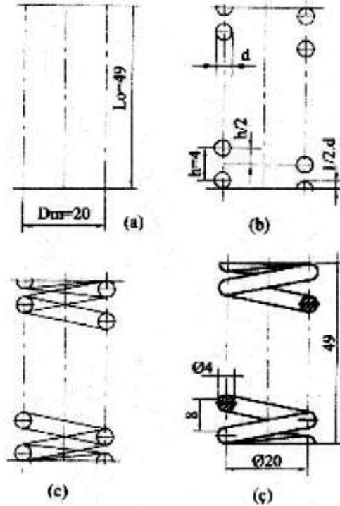
Şekil 2.11: Silindirik helisel yay çizmek
