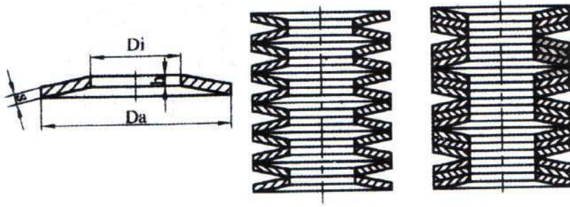
Şekil 2.5: Disk yaylar
