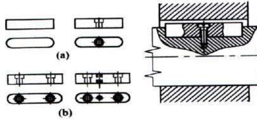
Şekil 1.10: Eğimsiz (Paralel yüzeyli) kalın (Takım tezgahları için) kamalar
