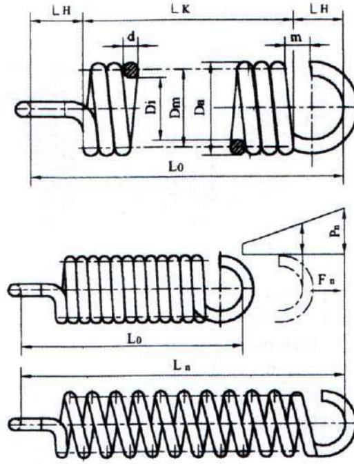
Şekil 2.3: Çekme yayı
