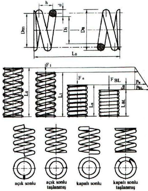
Şekil 2.2: Basma yayları
