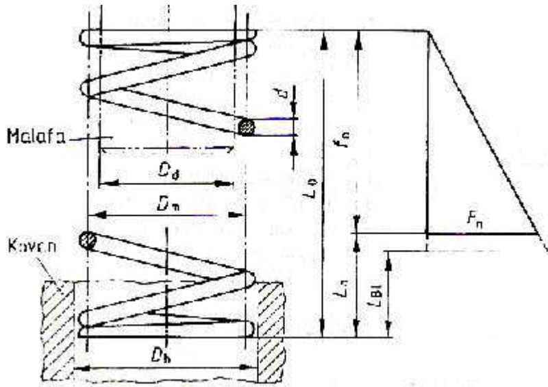
Şekil 2.10: Standart gösterilişleri
