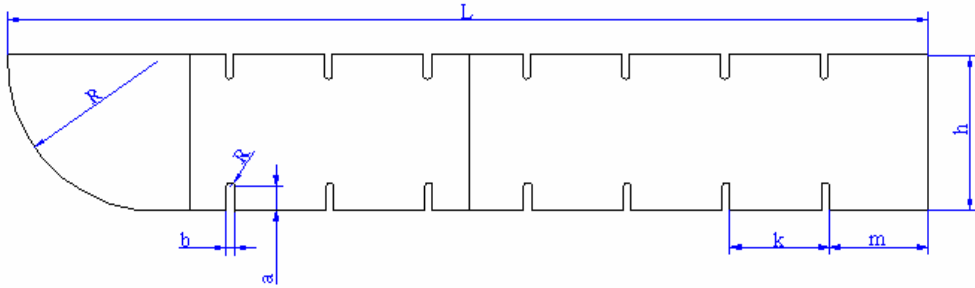
Şekil 2.6: Su geçirmez döşek imalat resmi
