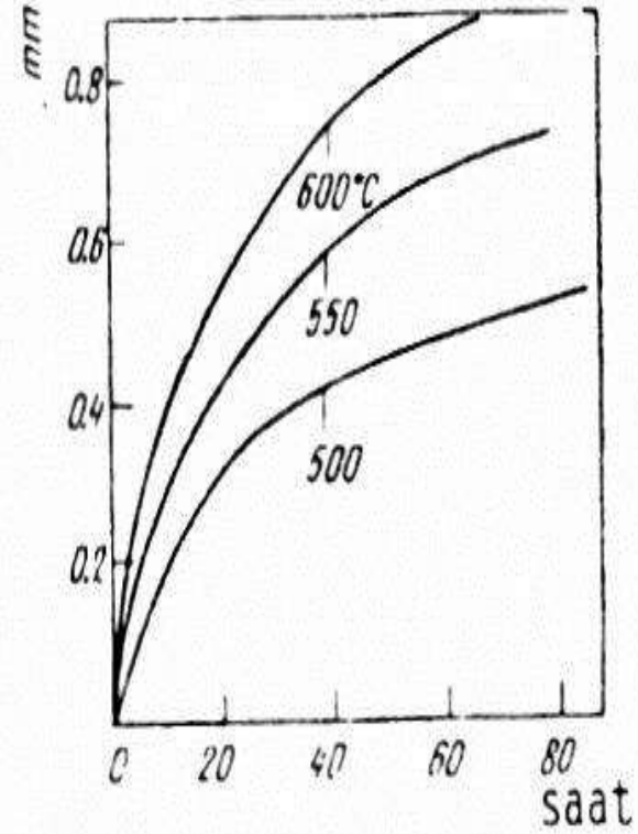
Nitrürasyon süresinin sert tabaka kalınlığına etkisi
